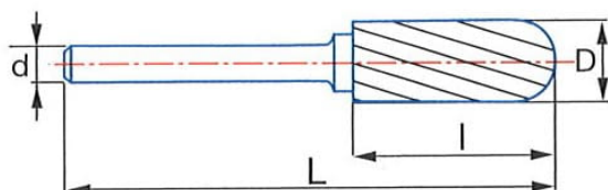
Fresa frontal radial
