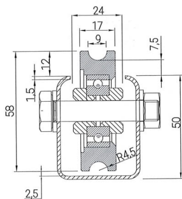
Esquema medidas rueda 60 mm
