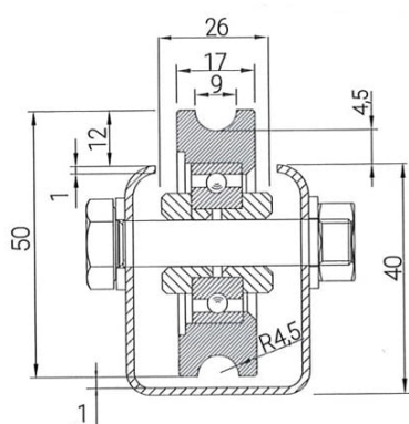
Esquema medidas rueda 50 mm
