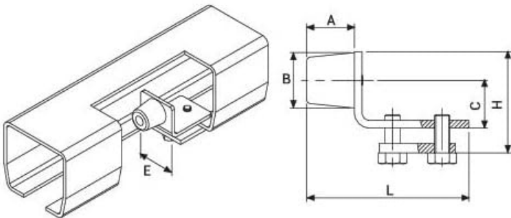
Medidas (mm)
