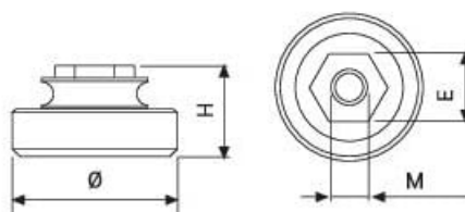
Medidas (mm)
