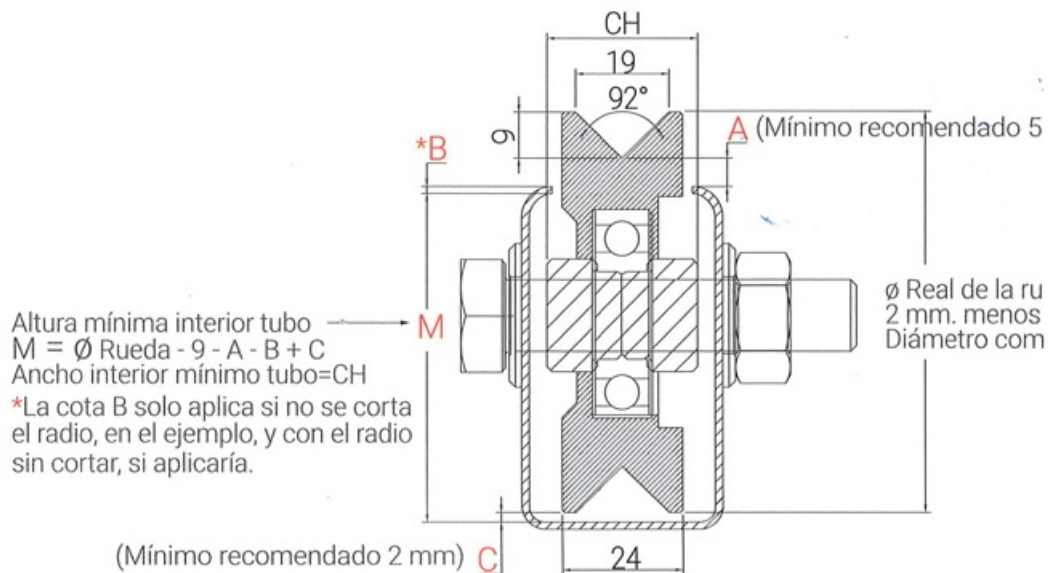
Medidas (mm)
