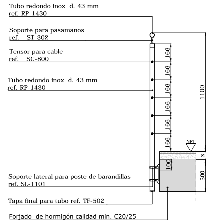
Sección A-A Barandilla R-Concept Easy Cable Montaje Lateral SL-1101 Escala 1:20
