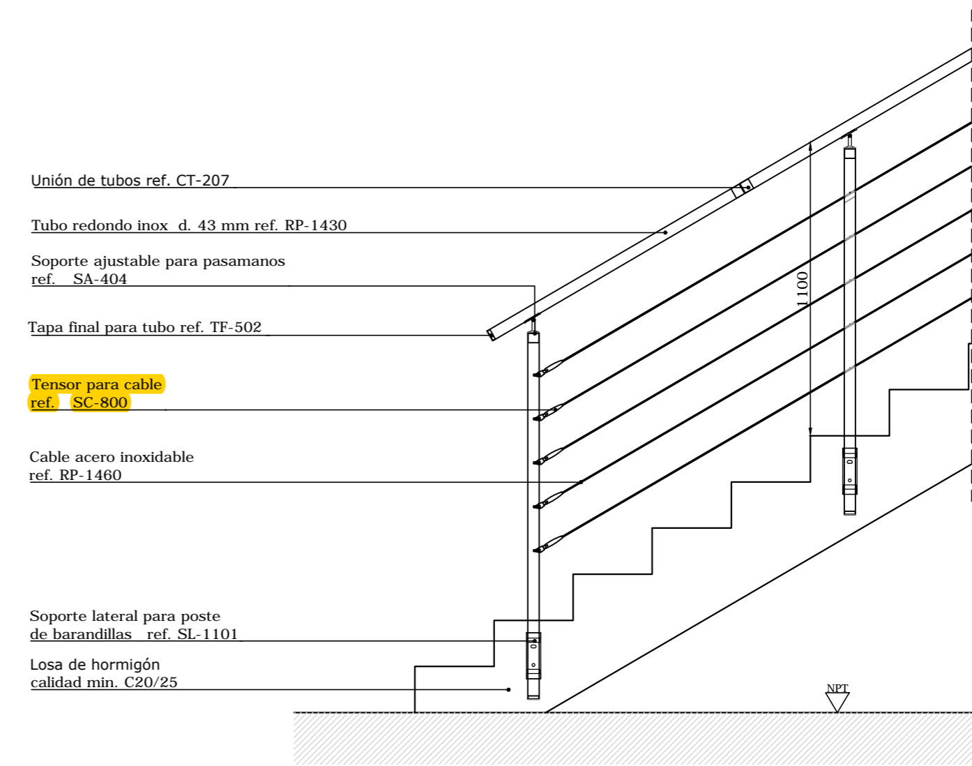
Detalle de arranque de escalera Barandilla R-Concept Easy Cable Montaje Lateral SL-1101 Escala 1:20
