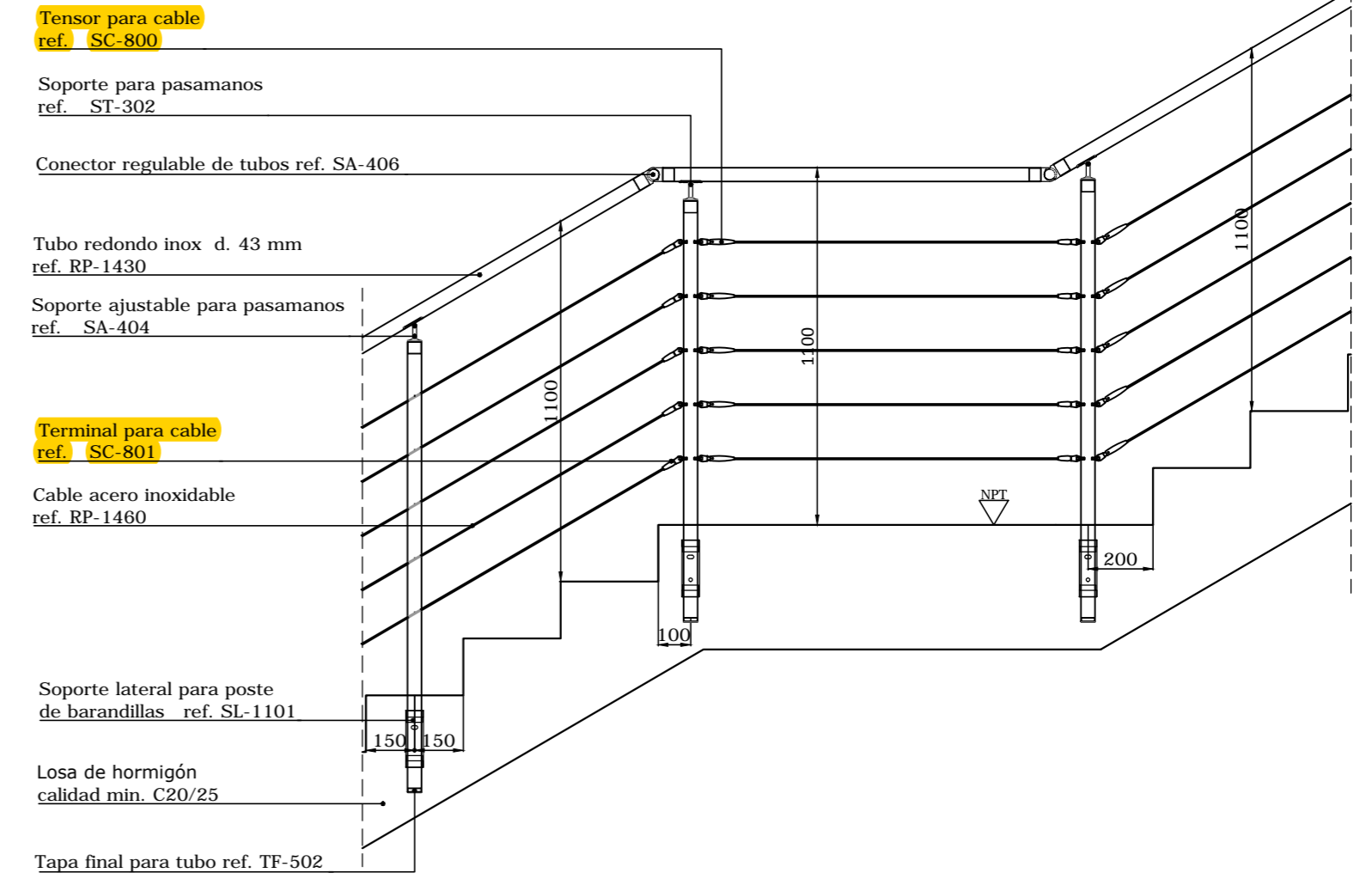
Detalle unión tramos inclinados con horizontal Barandilla R-Concept Easy Cable Montaje Lateral SL-1101 Escala 1:20
