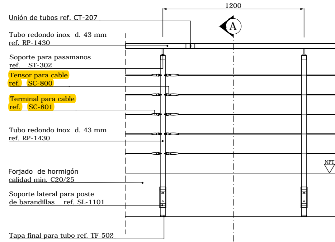
Detalle tramo horizontal tipo Barandilla R-Concept Easy Cable Montaje Lateral SL-1101 Escala 1:20
