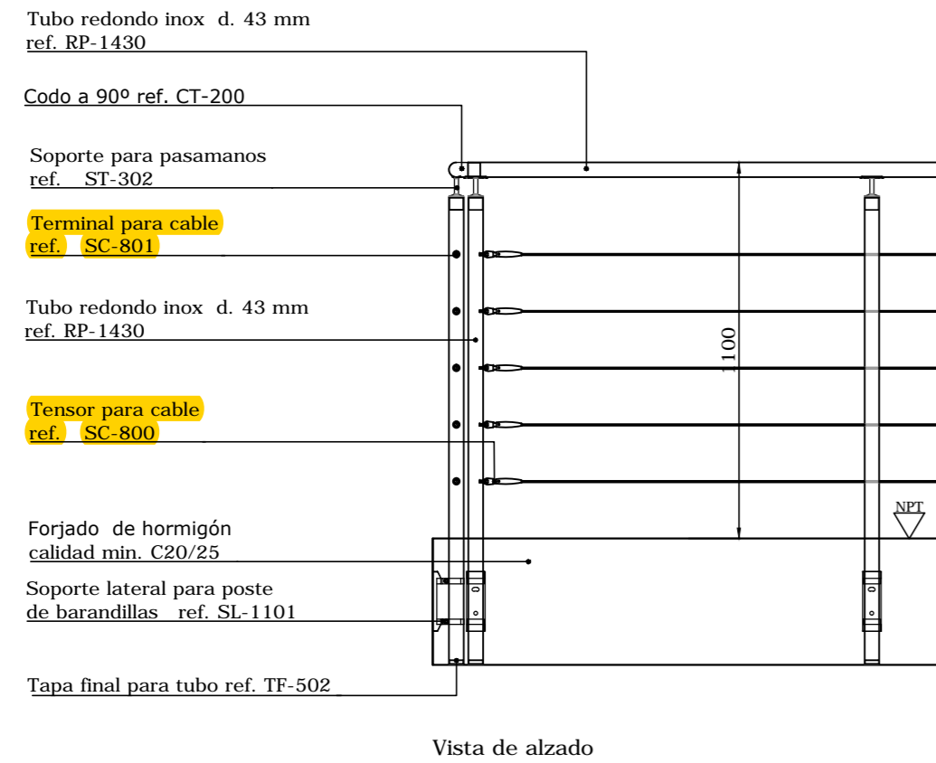
Vista de alzado
